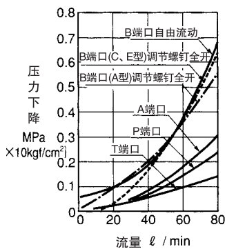
压力下降特性 MQ-03B-1※
