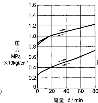
流量-压力特性 MQ-03B-1A
